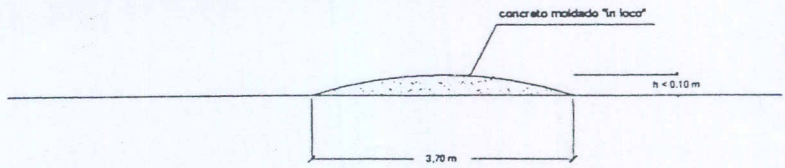
SEÇÃO TRANSVERSAL "TIPO II"
