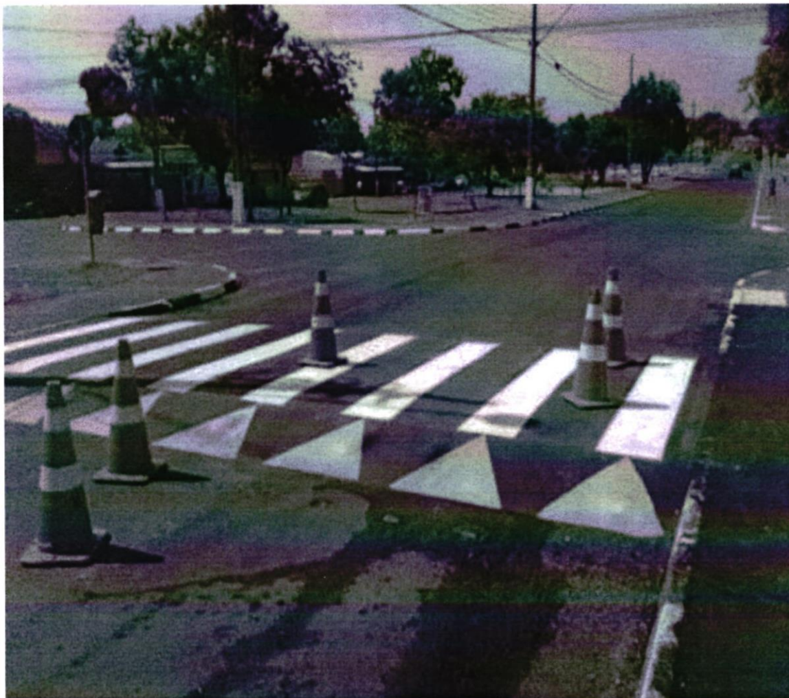
MODELO DE FAIXA ELEVADA.
